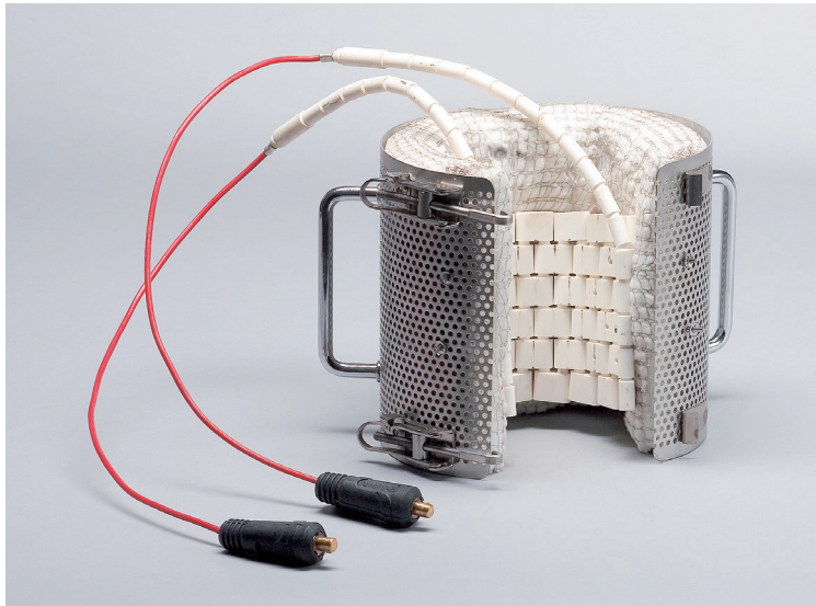
Akkor kelepçesi
