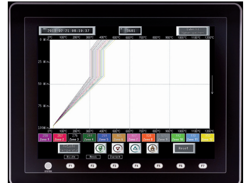
Sıcaklık/Zaman Diyagramı
