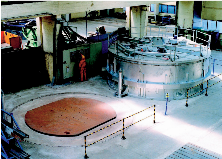
Elektrik ısıtmalı yuvarlak fırın İç çap: 6000 mm Açık yükseklik: 2000 mm Kurulu güç: 540 kW
